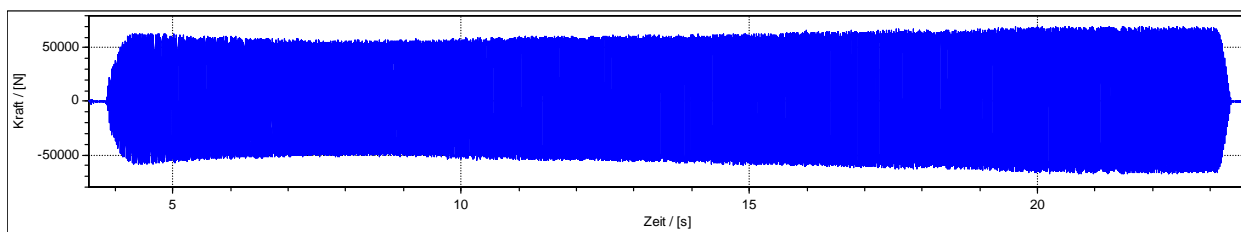
Abb.4: Kraftverlauf eines 36-96 Hz Sweeps auf einer bituminösen Tragdeckschicht mit autoadaptiver Kraftaussteuerung
